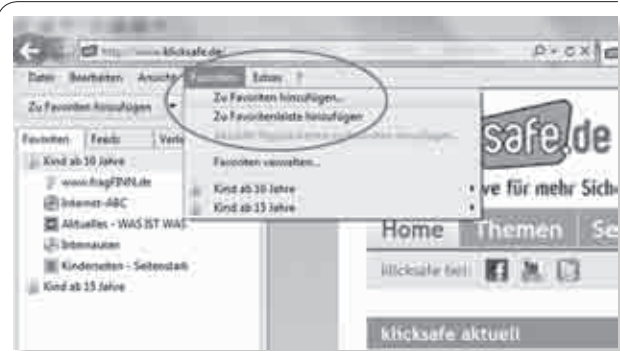
Favoriten einrichten
